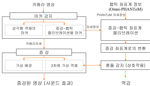
그림 2. 시스템 전체 알고리즘 흐름도
