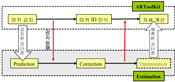
그림 5. 마커 감지 및 추적과 칼만 필터
